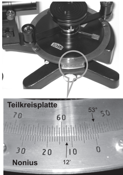
Abbildung 5: Die Spektrometer besitzen einen Nonius der den Winkel in Bogenminuten angibt. Das Ablesen geschieht folgendermaßen: Lesen Sie zunächst den Winkel der Teilkreis-skala mit dem Nullteilstrich des Nonius auf 0,5^\circ genau ab. Im unteren Bild beträgt der Winkel 53^\circ , da der Nullteilstrich zwischen 53^\circ und 53,5^\circ liegt. Die Nachkommastellen werden mit dem Nonius abgelesen. Beachten Sie, dass der Nonius in Bogenminuten geeicht ist. Dabei entsprechen die 30 Skalenteile (30' entspricht 30 Bogenminuten) einem halben Grad. Sie müssen nun den Teilstrich des Nonius suchen der genau unter einem Teilstrich der Kreisskala steht. Im Bild ist dies der Teilstrich 12. Das Ergebnis der Winkelmessung ist demnach 53^\circ 12' bzw. im Gradmaß: 53^\circ + (12'/60') = 53,2^\circ .
