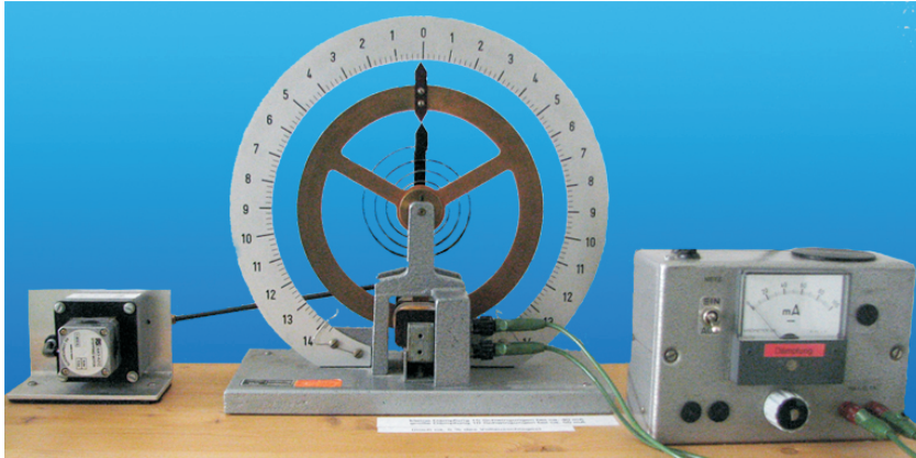
Abbildung 1: Versuchsaufbau
